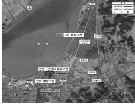
지중화 노선도
